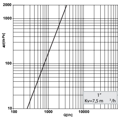
Curva de pérdida de carga
